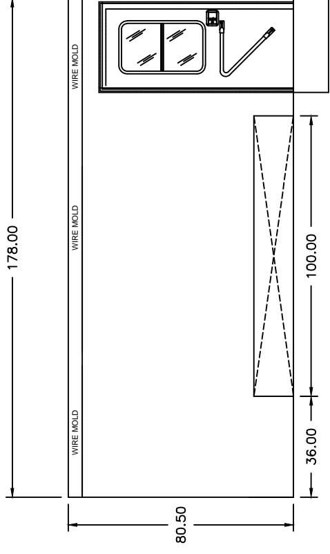
CURBSIDE WALL
